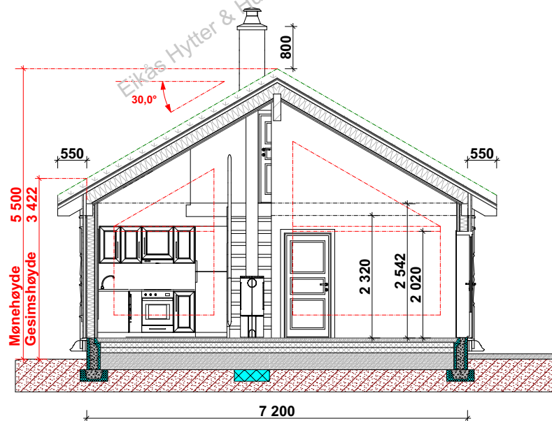
Snitt A-A
