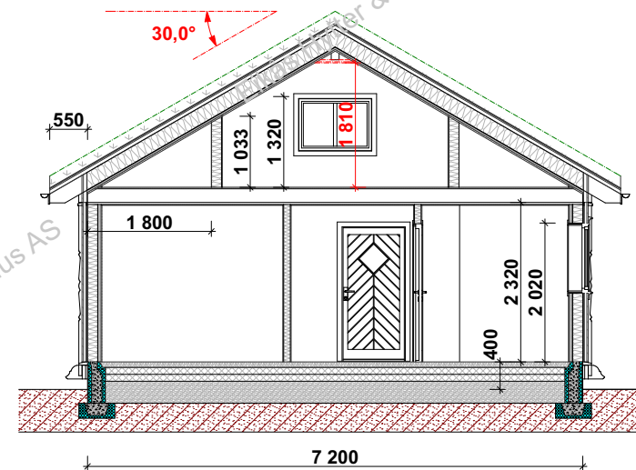
Snitt B-B
