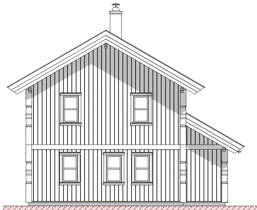
Fasade 1
