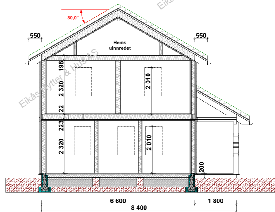
Snitt B-B
