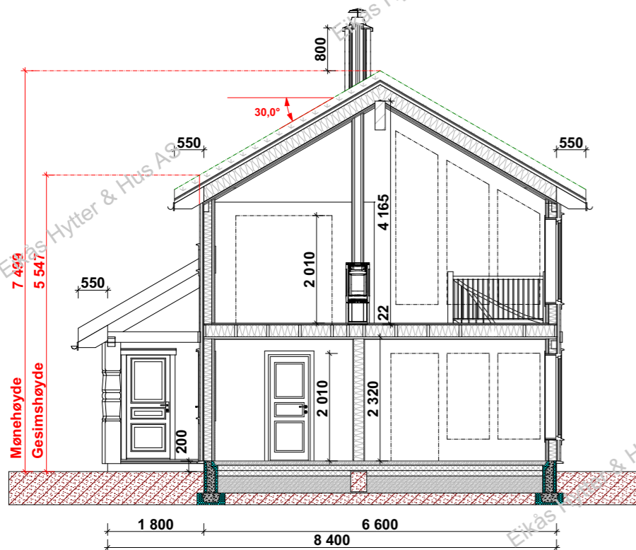
Snitt A-A
